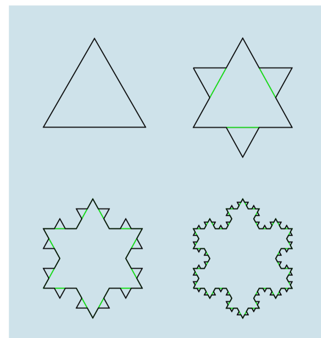
"KochFlake". Licensed under CC BY-SA 3.0 via Wikimedia Commons http://commons.wikimedia.org/wiki/File:KochFlake.svg#/media/File:KochFlake.svg
